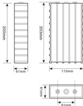
型号(MODEL): TS-LYP60AHA
